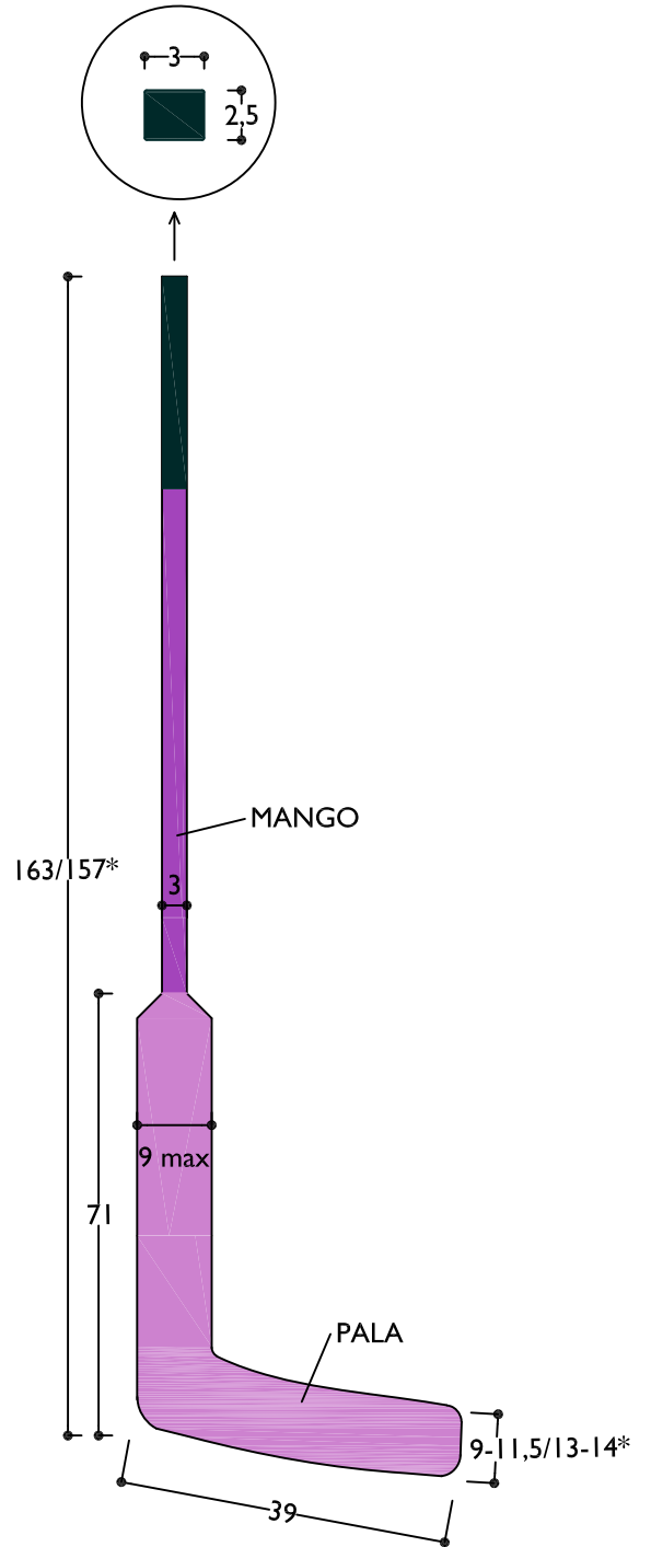
PALO O "STICK" DEL PORTERO
