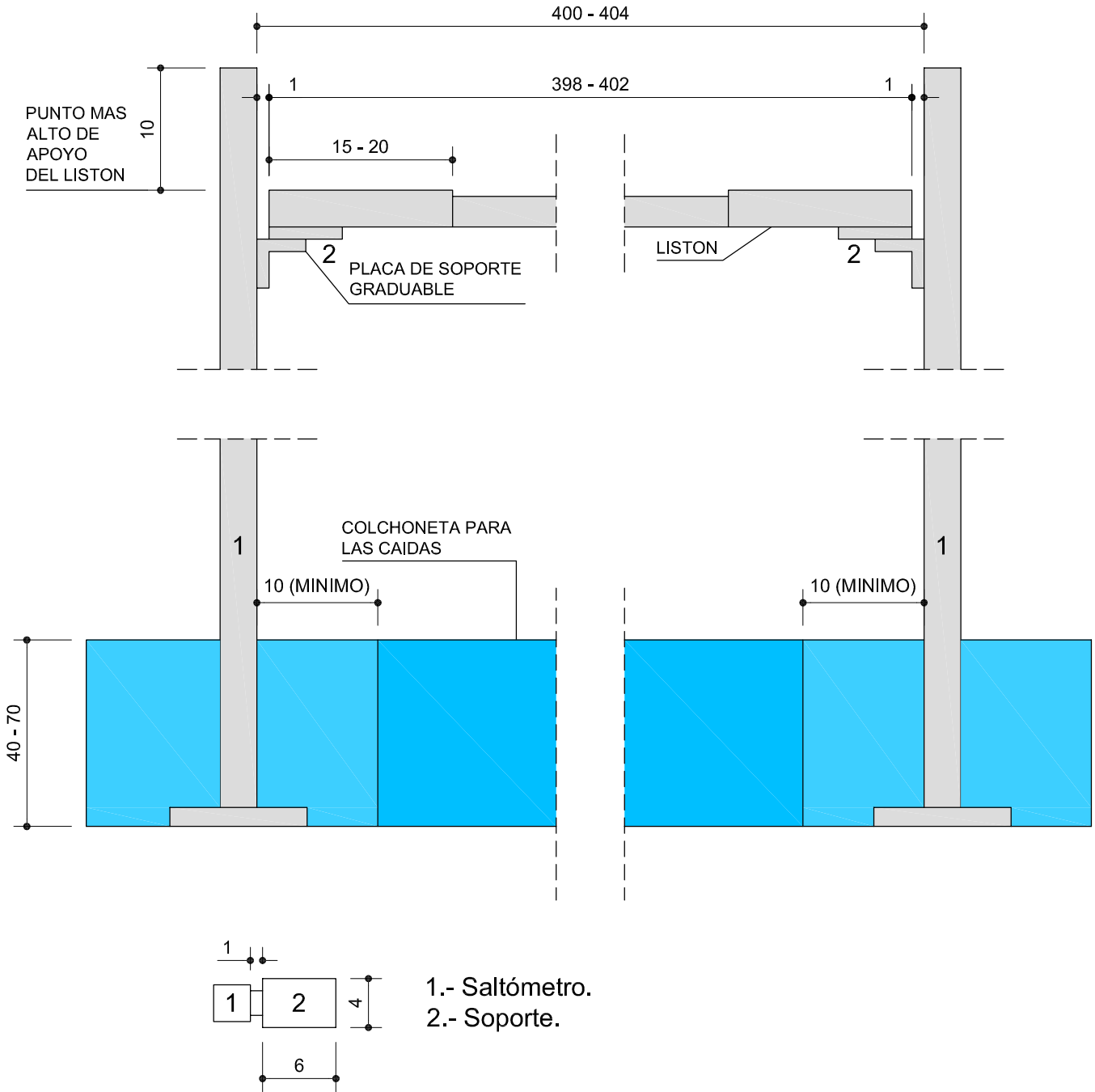
SOPORTE (PLANTA)
