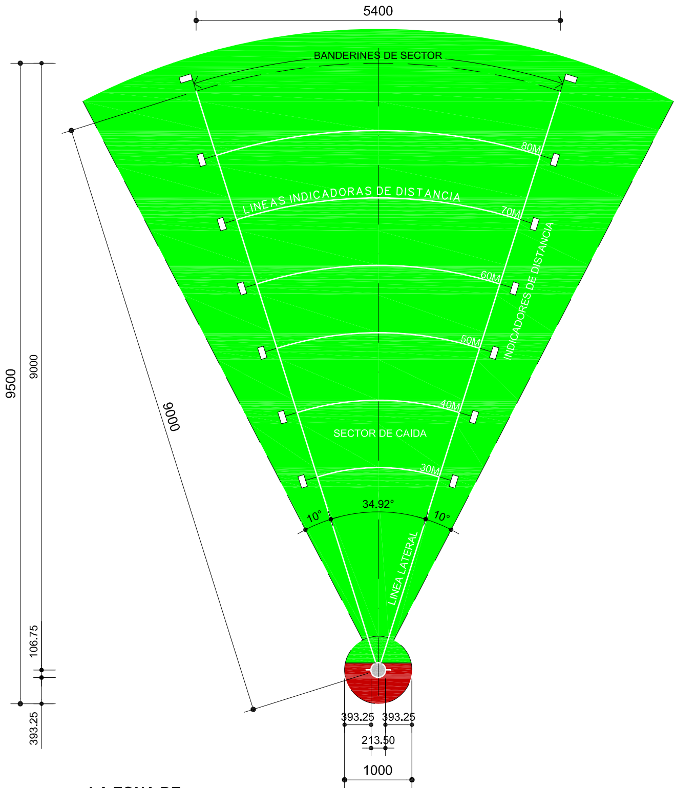
LA ZONA DE LANZAMIENTOS ATLm-1
