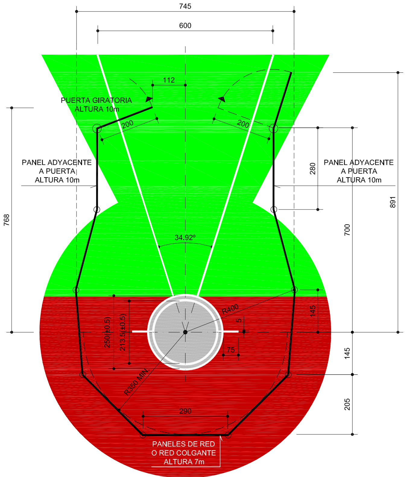
JAULA PARA MARTILLO Y DISCO CON CIRCULOS CONCENTRICOS ATLm-9a
