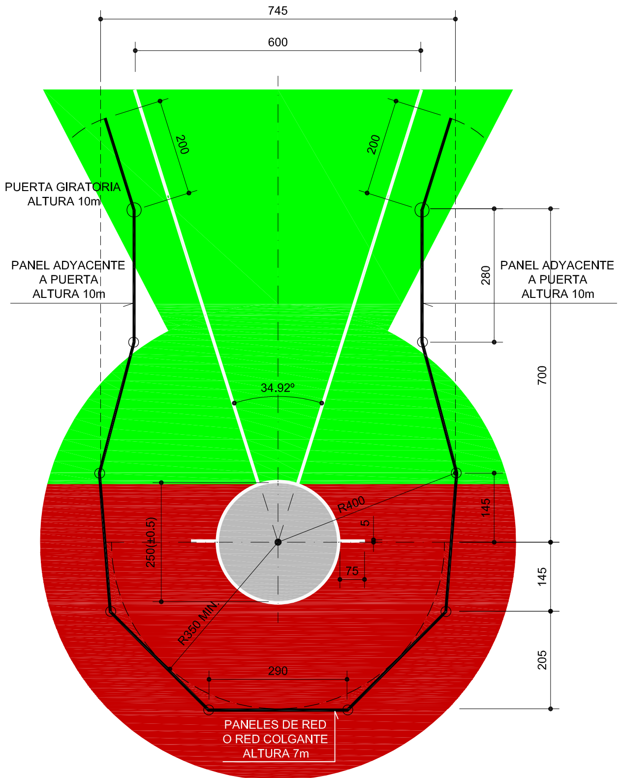
JAULA PARA MARTILLO Y DISCO EN CONFIGURACION DE DISCO ATLm-9b
