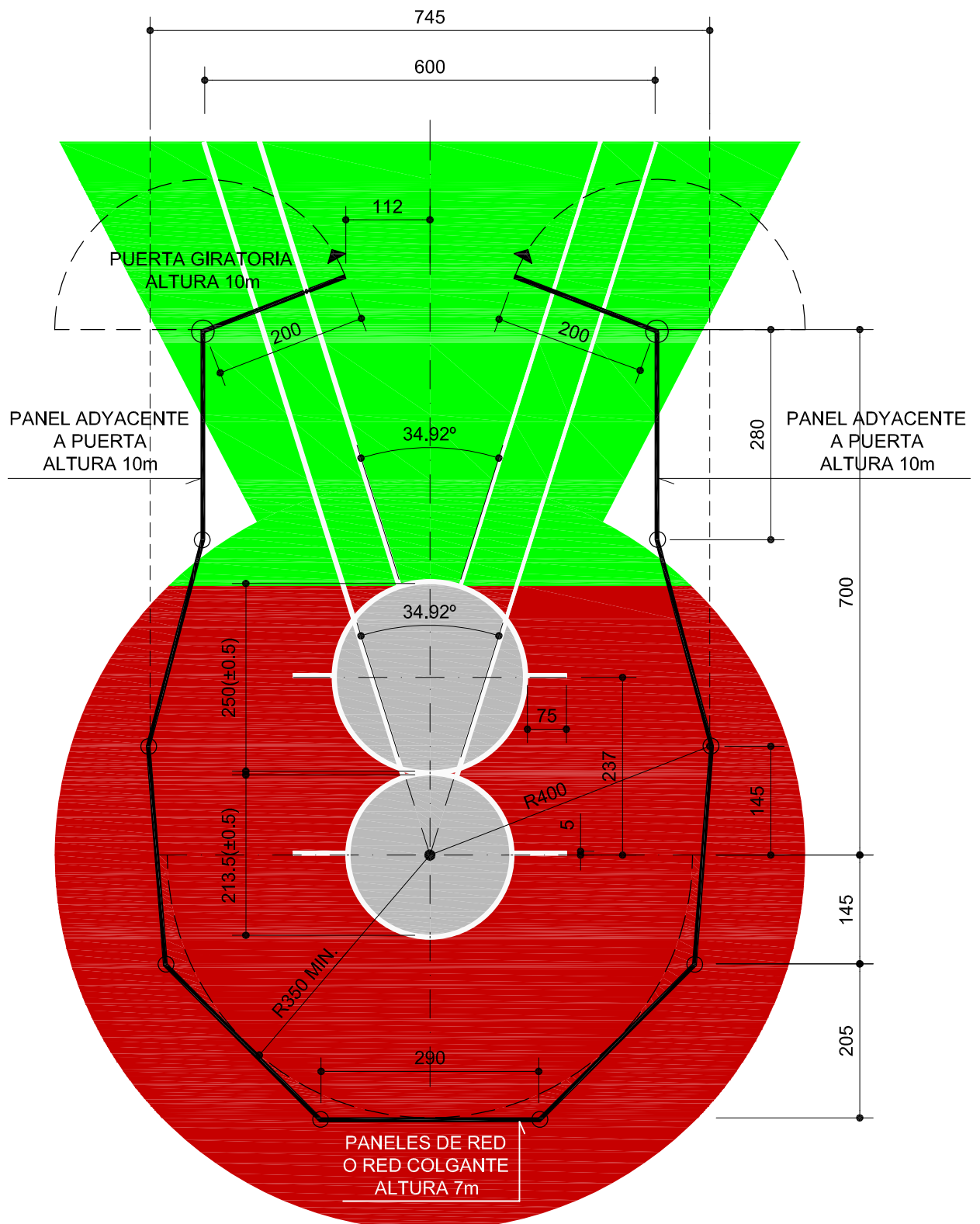
JAULA PARA MARTILLO Y DISCO CON CIRCULOS INDEPENDIENTES ATLm-9c
