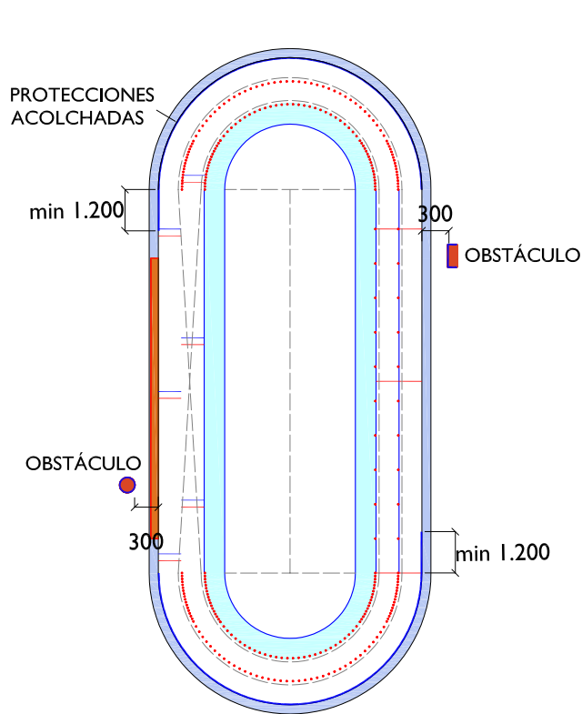
DISPOSICIONES MÍNIMAS: Protecciones en curvas + 12 m Frente a obstáculos a menos de 3 m.
