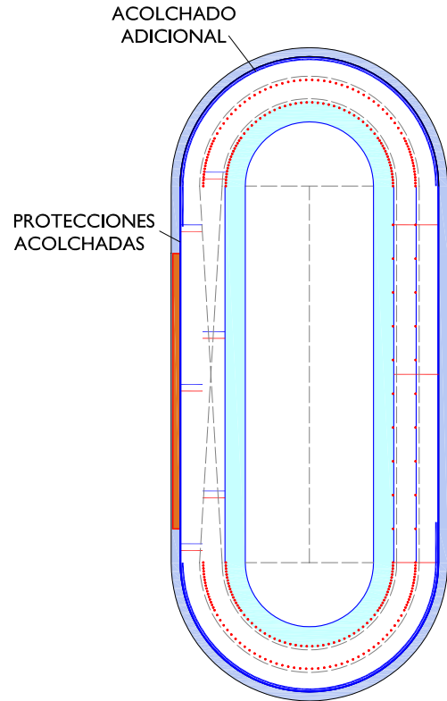
JUEGOS OLÍMPICOS Y COMPETICIONES DE LA ISU: Protecciones en todo el perímetro y acolchado adicional en curvas
